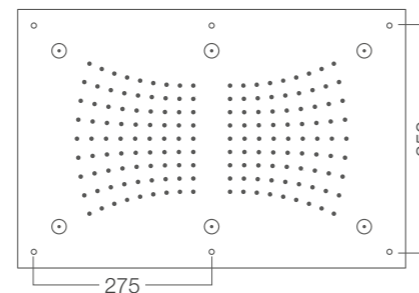
KI 221 / KI 261 ✓ L 600x400 mm ✓ G. 1/2" M
