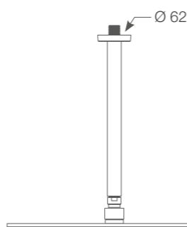
LA 804 □ 400x400 mm ✓ H 357 mm ✓ G. 1/2" M
