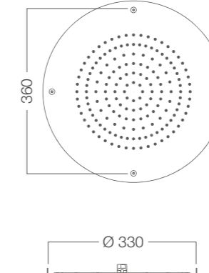
KI 012 ✓ Ø 400 mm ✓ G. 1/2" M
