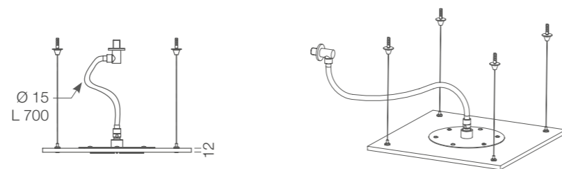
CR 001 □ 450x450 mm ✓ G. 1/2" M
